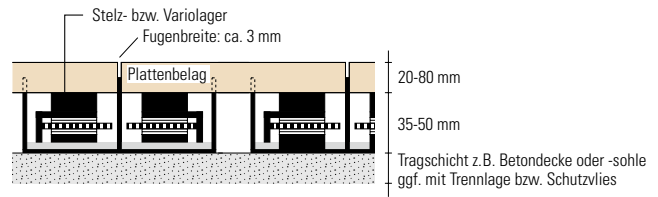
Plattenverlegung auf Stelzlagern (Fugen offen)
